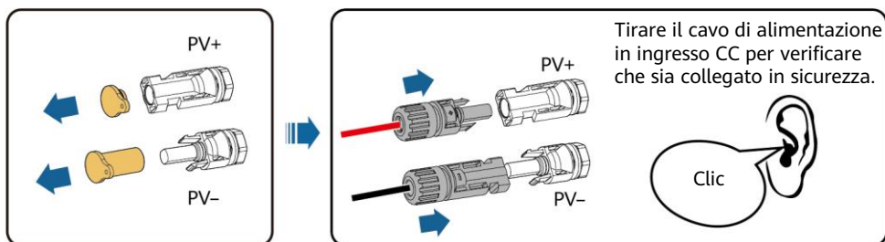
Terminali di ingresso CC
