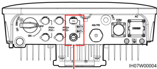
Terminali batteria (BAT+/BAT-)
